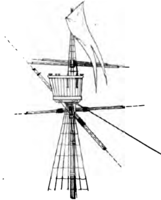
ΕΙΚ. 87. Ἄτερον εἶδος Ἑλληνικοῦ καρχήσιου κατὰ τὸν Μῆσαιῶνα, μετὸν διὰ τοὺς μαχητὰς χώρον — τὸ πολέμιστρον — πρὸς τὰ ὀπίσω.
