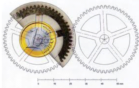
Το Γρανάζι της Σαρδηνίας με εμφανή την καμπυλότητα οδόντωσης
